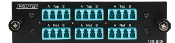
3-Link 40G BiDi TAP
